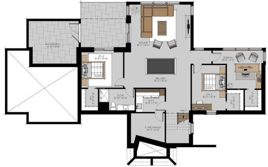
PLAN DU SOUS-SOL 1611 PI.CA.
