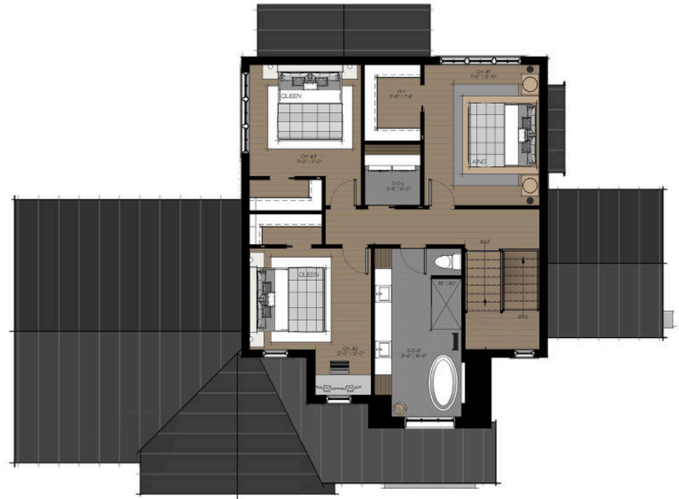
PLAN DE L'ÉTAGE 996 PI.CA.
