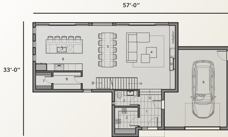
PLAN DU REZ-DE-CHAUSSÉE 1039 PI.CA.
