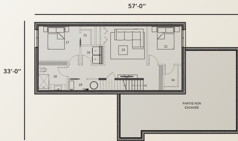
PLAN DU SOUS-SOL (optionnel) 840 PI.CA.
