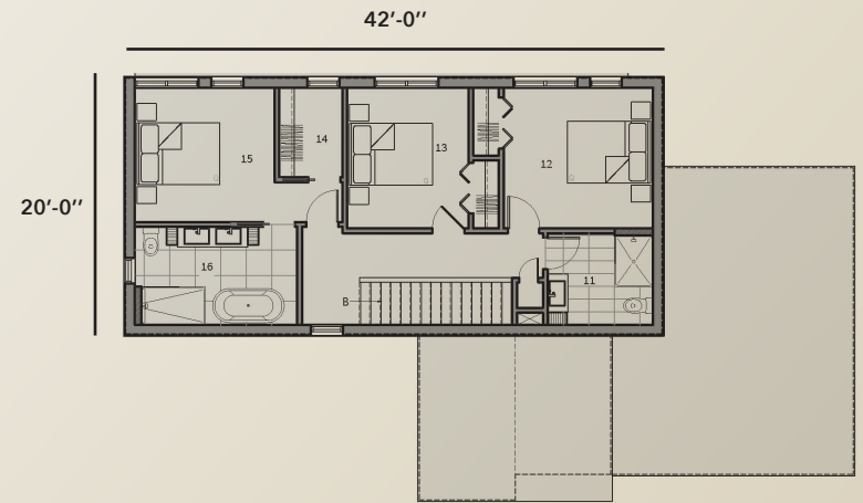
PLAN DE L'ÉTAGE 856 PI.CA.
