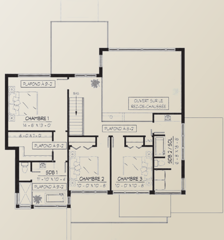
PLAN DE L'ÉTAGE 1 078 PI.CA.
