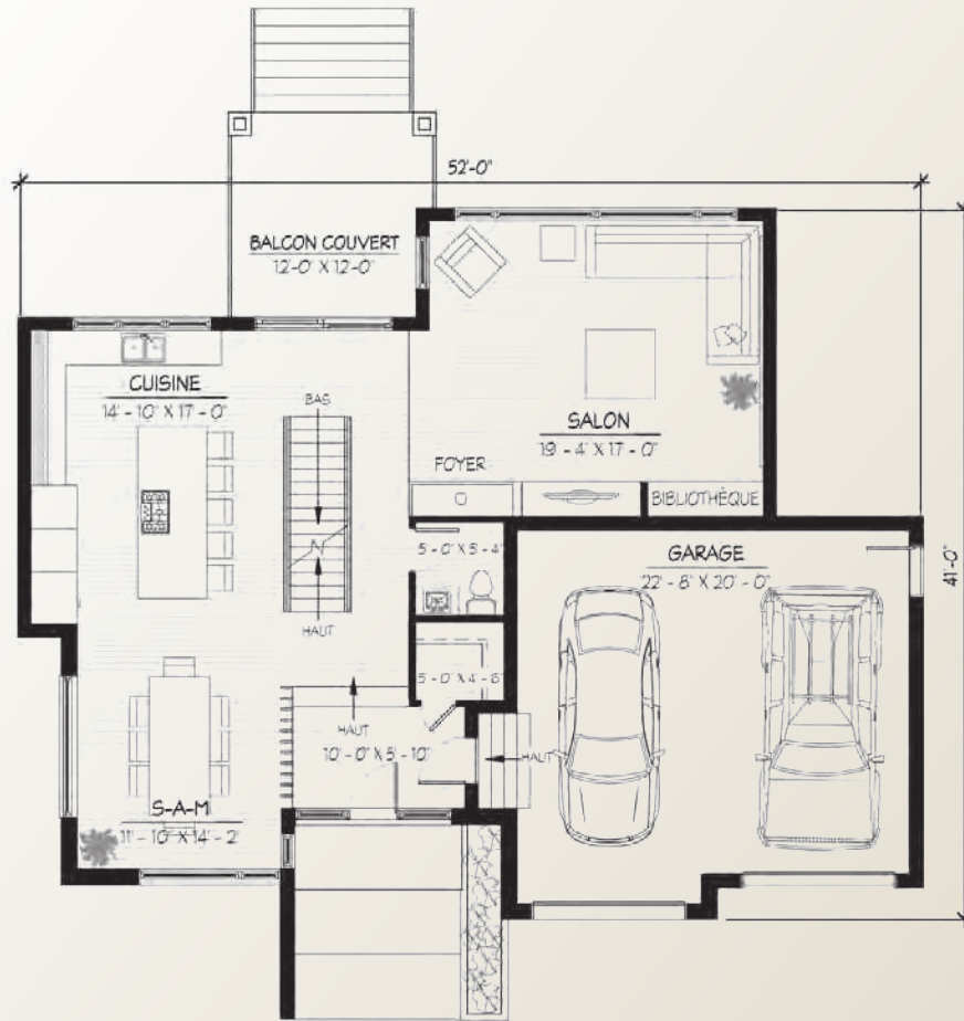
PLAN DU REZ-DE-CHAUSSÉE 1 144 PI.CA.
