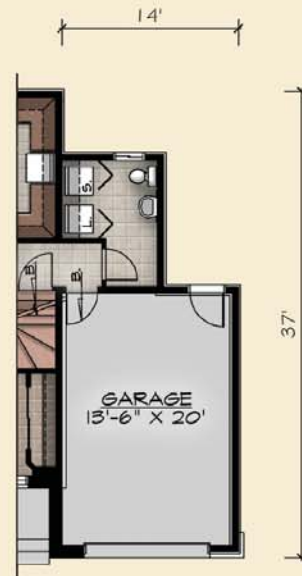
PLAN DU REZ-DE-CHAUSSEE GARAGE SUP.: 310 pl.ca. (SANS SALLE DE CINEMA)
